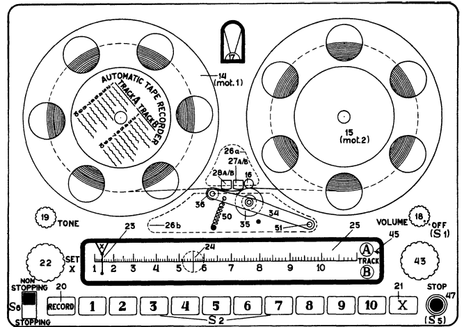
Rechts: Bild 10. Entwurf für die Deckplatte eines Tonband-Automaten nach der US-Patentanmeldung 721.599
