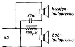
Bild 4. Schaltung der Grundig-Raumklang-Box II
