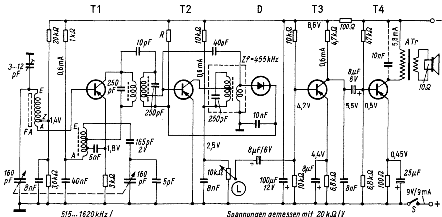
Bild 2. Taschensuper Rexetta mit Reflexschaltung
