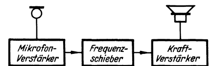
Schaltung eines Frequenzschiebers zwischen Mikrofon- und Kraftverstärker zur Vermeidung akustischer Rückkopplung
