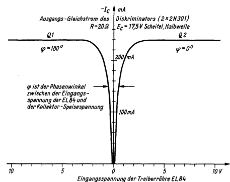
Bild 8. Richtstrom-Kennlinie des Phasendiskriminators
