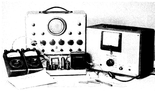
Bild 7. Messplatz zur Untersuchung des Phasen-Diskriminators
