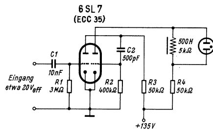
Schaltung eines Gerätes zur Erzeugung kurzer Lichtblitze in der Folge der Eingangsfrequenz
