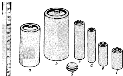
Bild 3. Verschiedene Typen von Rundzellen; a = Babyzelle, b = Monozelle, c = Mignonzelle, d = Mikrozelle, e = Ladyzelle, f = halbe Mignonzelle, g = Knopfzelle. Diese Knopfzelle hat die gleichen Abmessungen wie eine entsprechende Deacelle und kann daher ersatzweise für solche Deacellen benutzt werden
