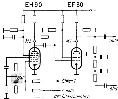
Bild 1. Die Schaltung des Amplitudensiebes mit dem schadhaft gewordenen Kondensator
