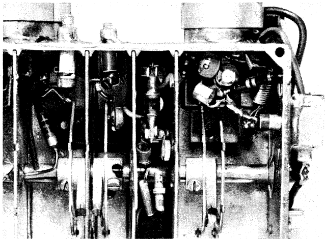
Bild 5. Blick in die offenen Kammern des Tuners; links das zweikreisige Bandfilter mit der Messingzwischenwand, in der Mitte die Mischstufe mit der UHF-Siliziumdiode und rechts der Oszillatorteil mit außen angebaute Vormagnetisierungseinheit
