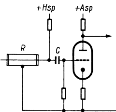
So kann ein Stück Koax-Kabel (C) zur Ankopplung des Geiger-Müller-Zählrohres (R) verwendet werden
